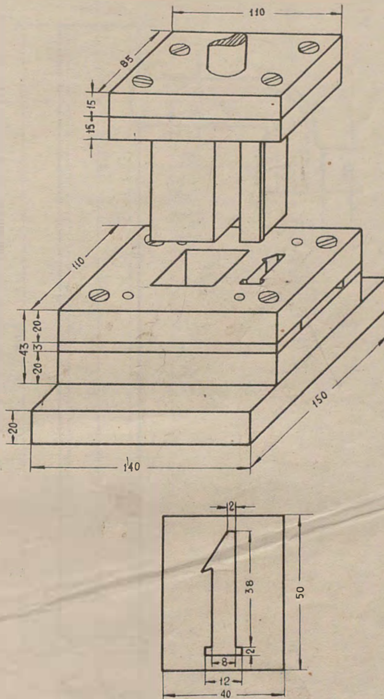
10.º—Chapa de numeración.—Macho y hembra.
