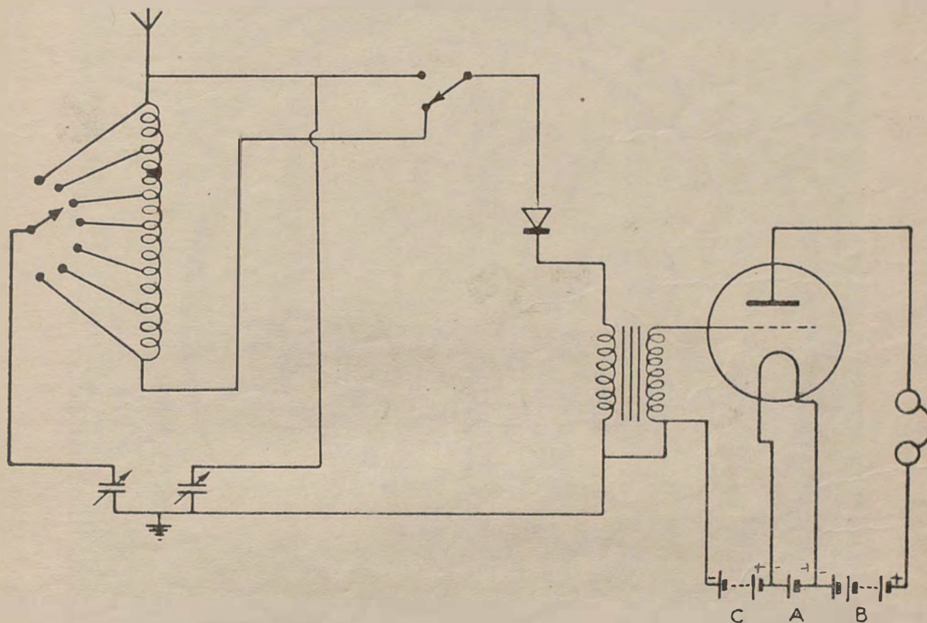
6.º—Receptor de galena con paso de amplificación en baja frecuencia.
