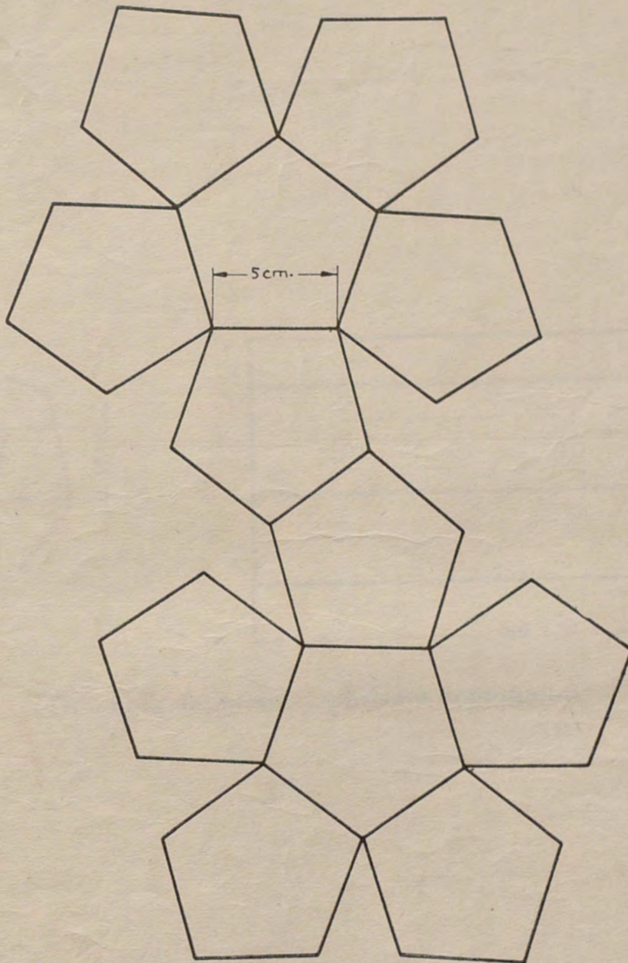
13.º—Dodecaedro con chapa de cinc corriente.
