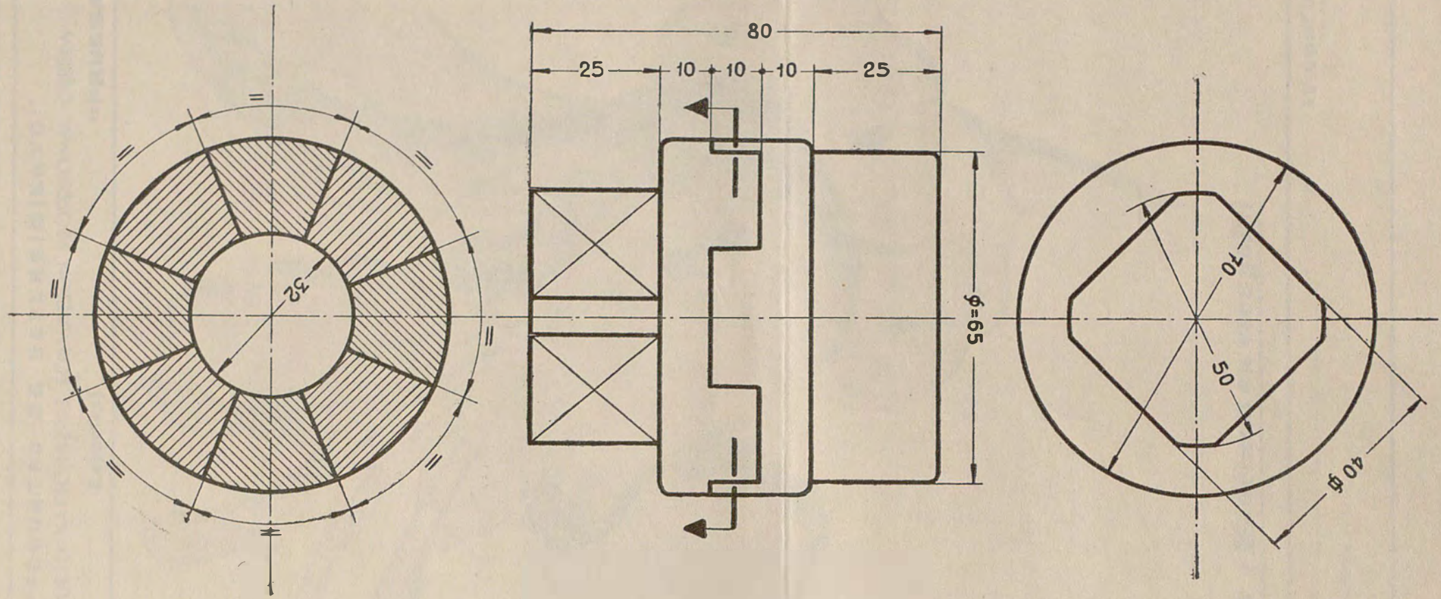
Machón de embrague
