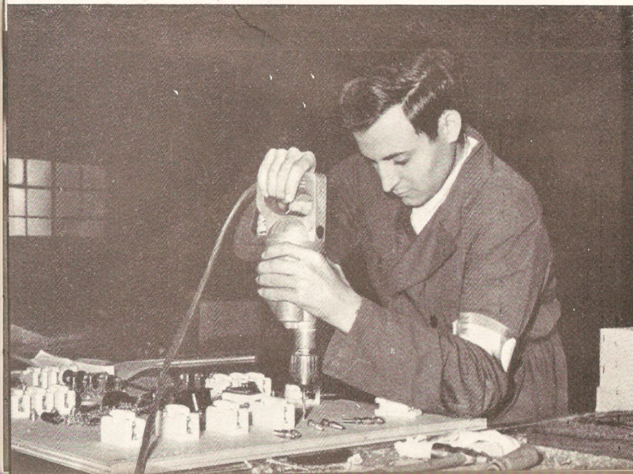
Un aprendiz de montador prepara su cuadro de distribución en uno de los Concursos Laborales.
