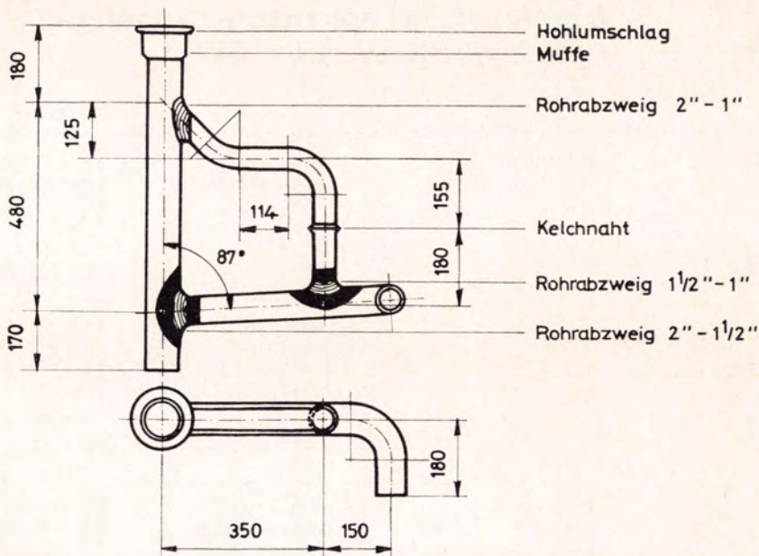
Beispiel einer Wettbewerbsaufgabe für Spengler-Installateur, Bleirohrarbeiten
